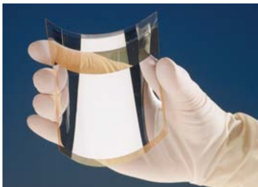
Cellule solaire plastique souple de grande dimension (100 mm × 100 mm) fabriquée au Genec.
